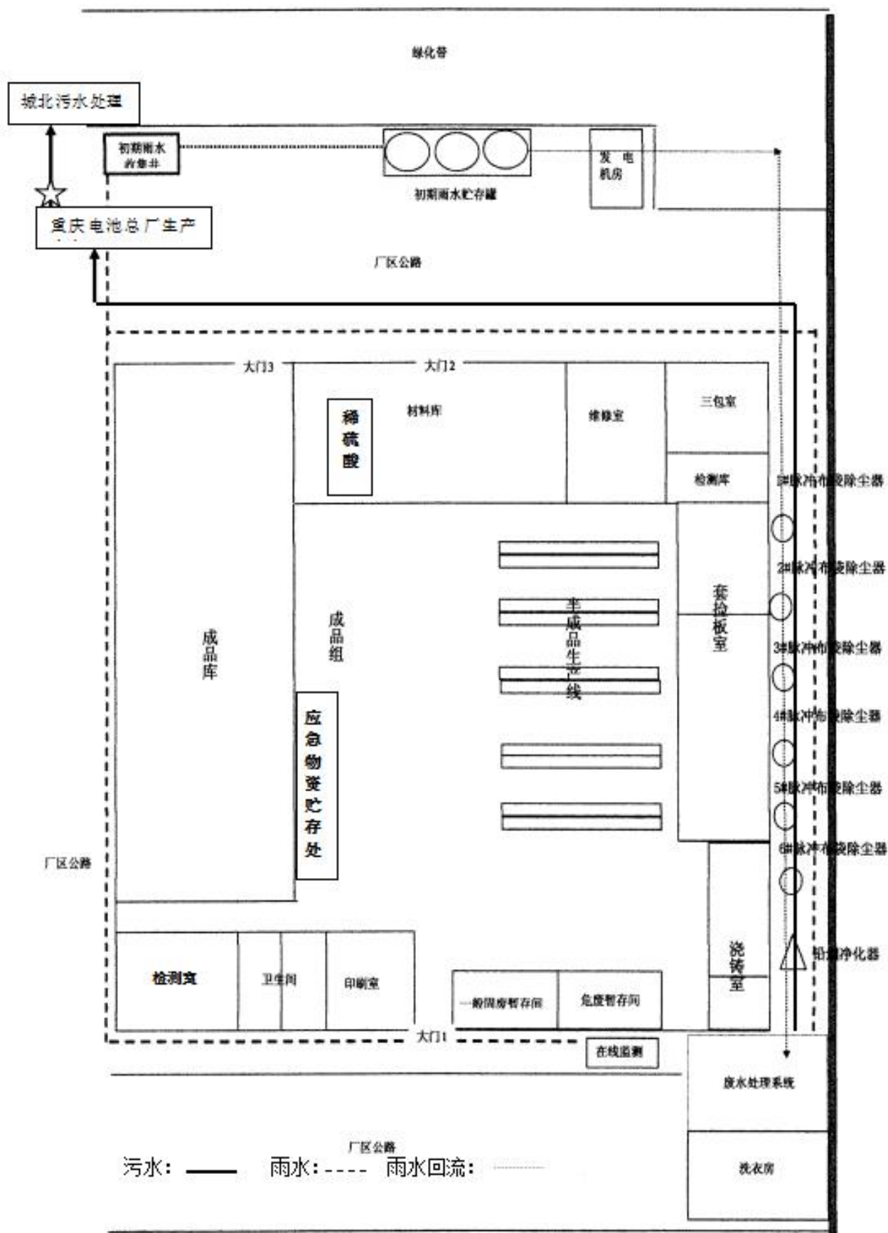
附图 4：厂区平面布置及雨污管网图
